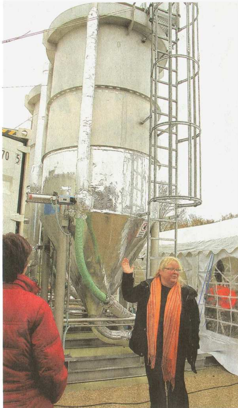
Susanne Kimmich (rechts), technische Leiterin der Firma Epuramat, zeigt die beiden ExSep-Silos, so der Name der Reinigungsanlage, in denen das Wasser vorgeklärt und von Sand und Fett befreit wird. Foto: Manfred Dittenhofer
